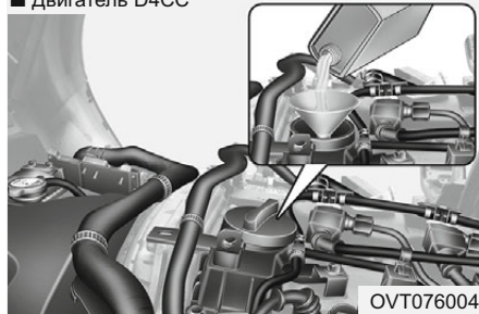
■ Двигатель D4CC
