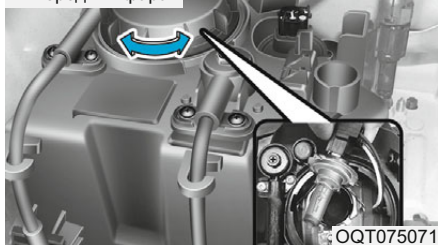
■ Передняя фара
