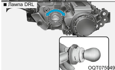
■ Передняя фара
