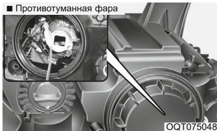
■ Лампа DRL
